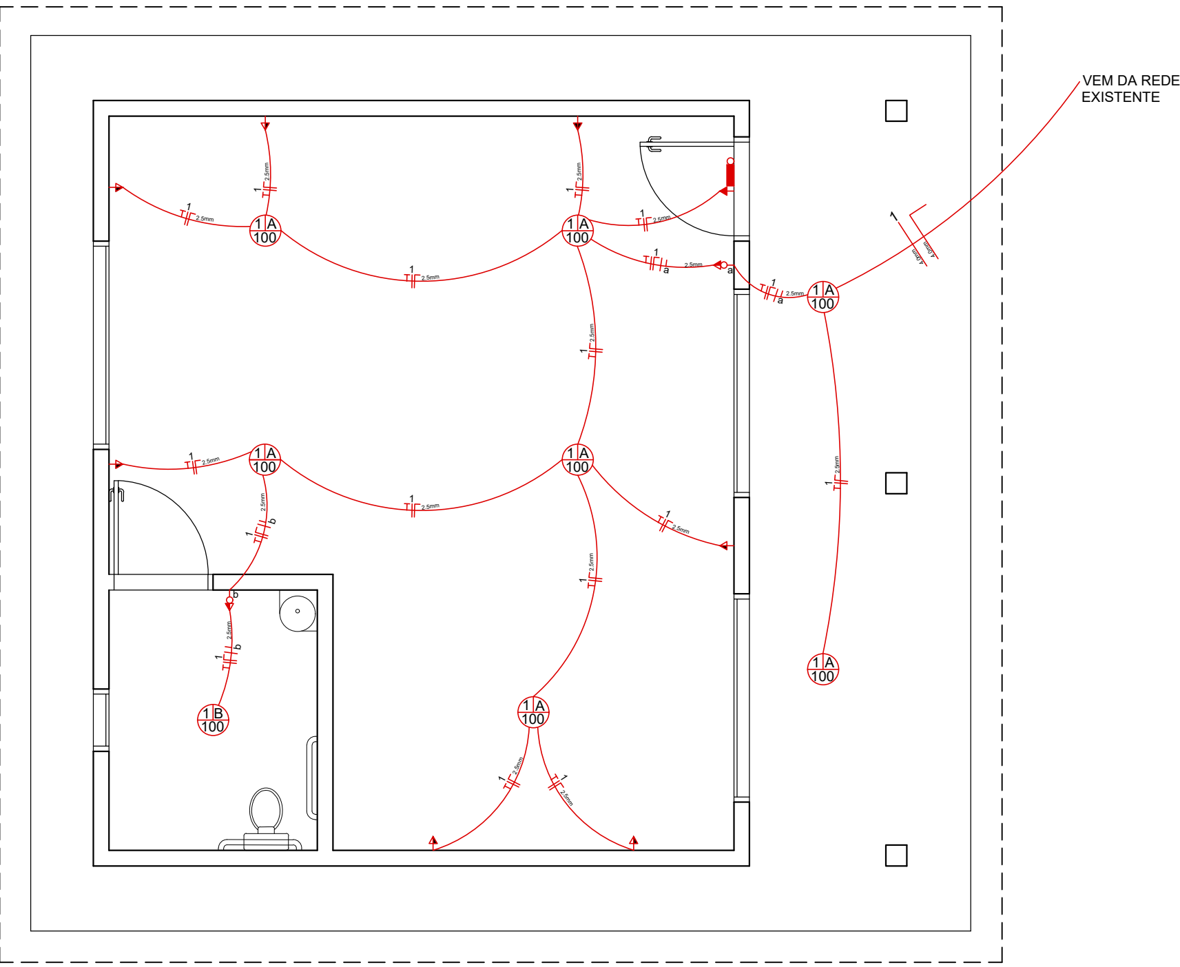
PROJETO ELÉTRICO ESC.: 1/50
