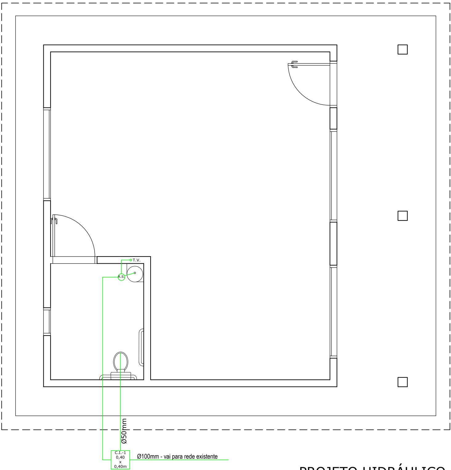
PROJETO HIDRÁULICO ESC.: 1/50
