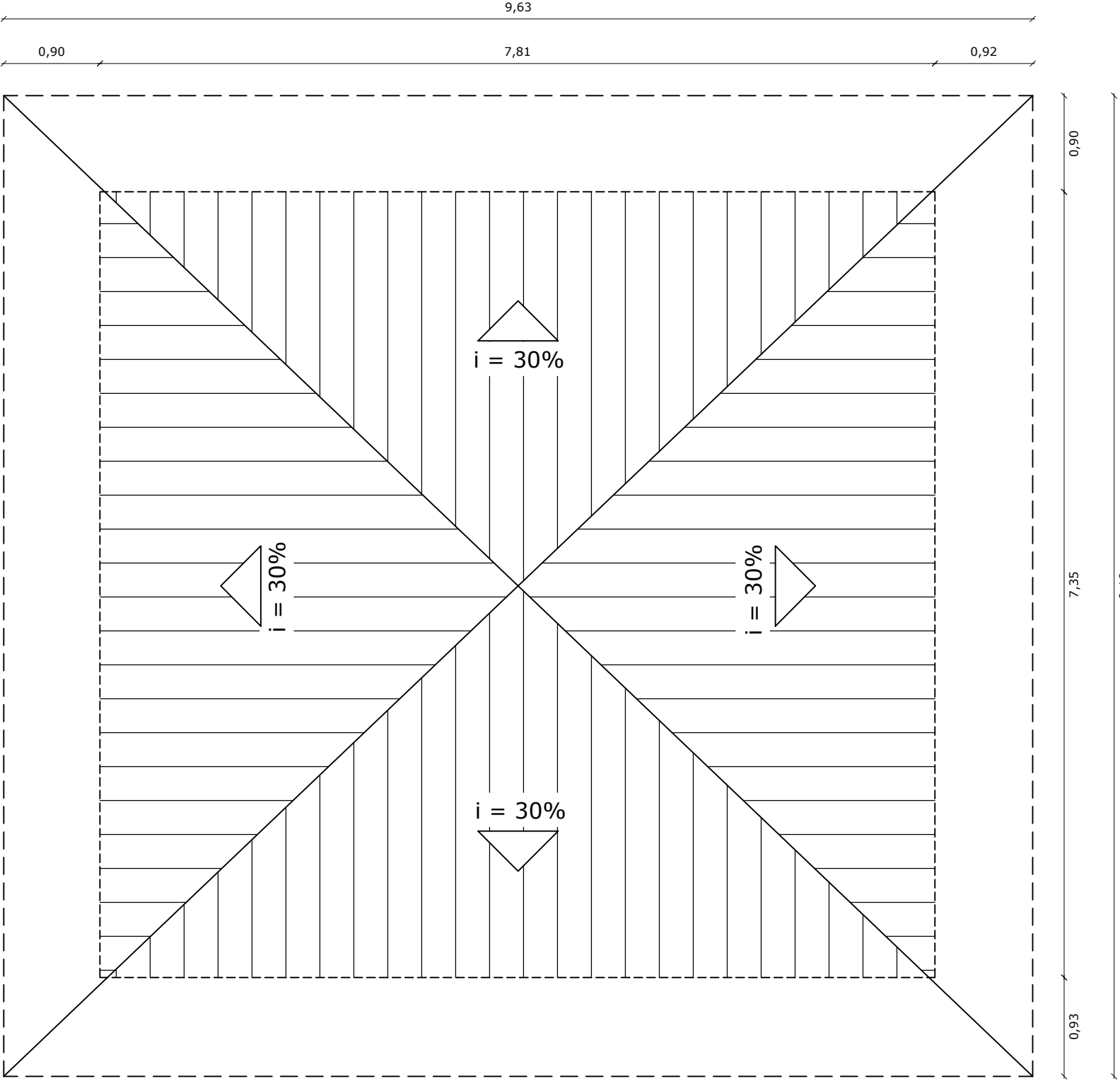
PLANTA COBERTURA ESC.: 1/50
