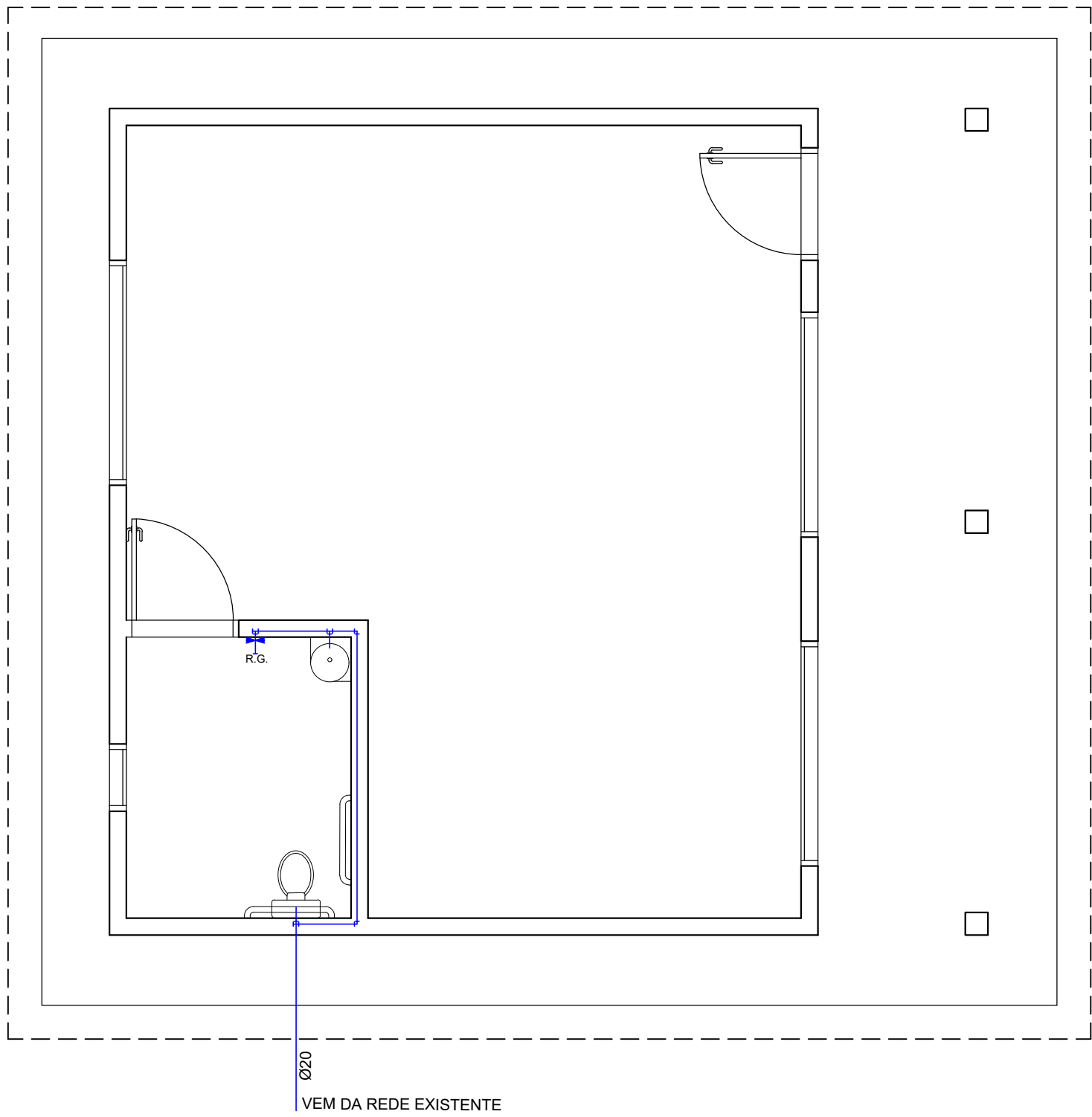
PROJETO HIDROSSANITÁRIO ESC.: 1/50
