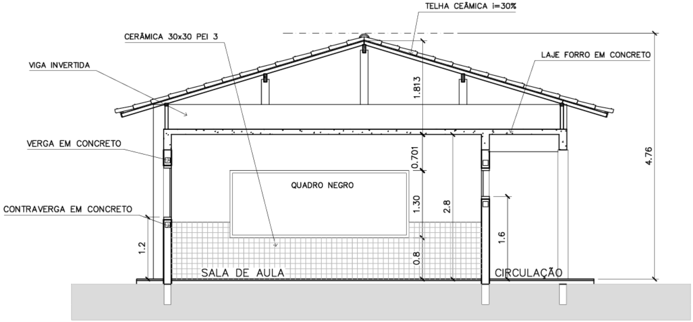
CORTE ESQUEMÁTICO
